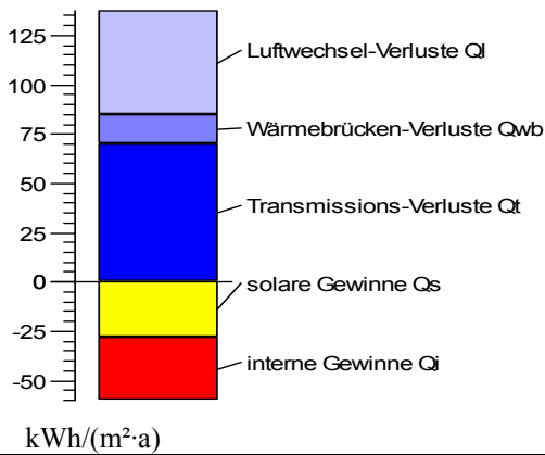
Energiebilanz Q''_H
