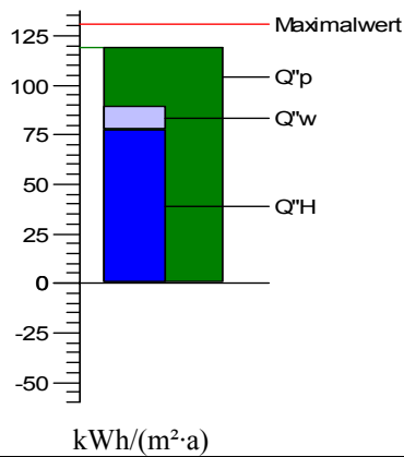
Primärenergie Q''_p
